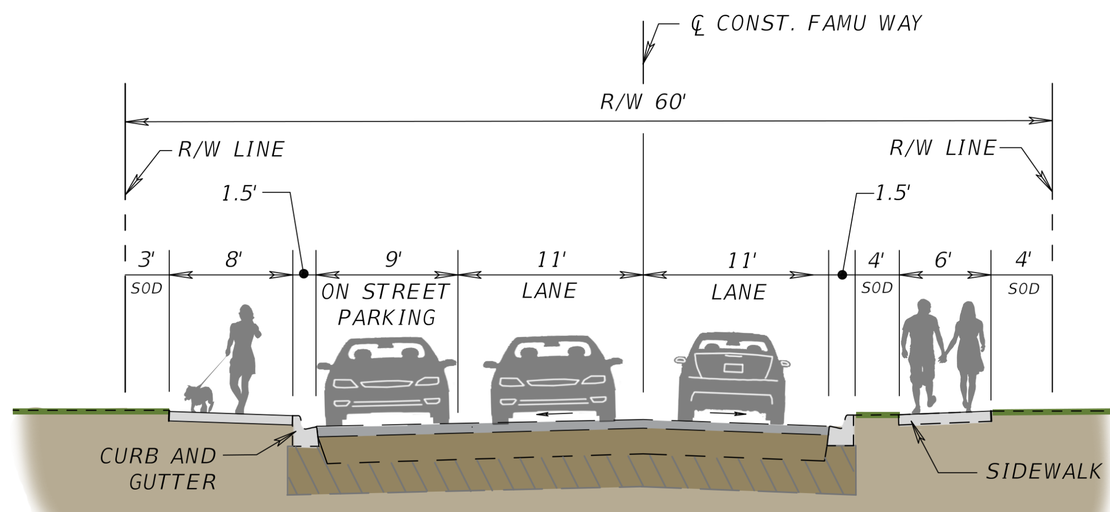
SECTION A-A'
